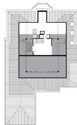
Tweede verdieping
