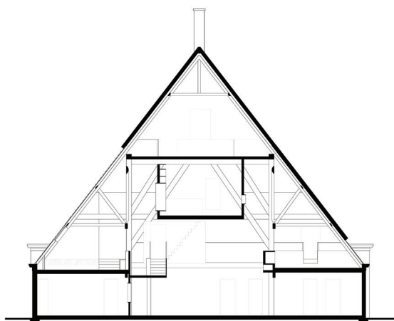
Doorsnede
