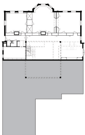
Begane grond
