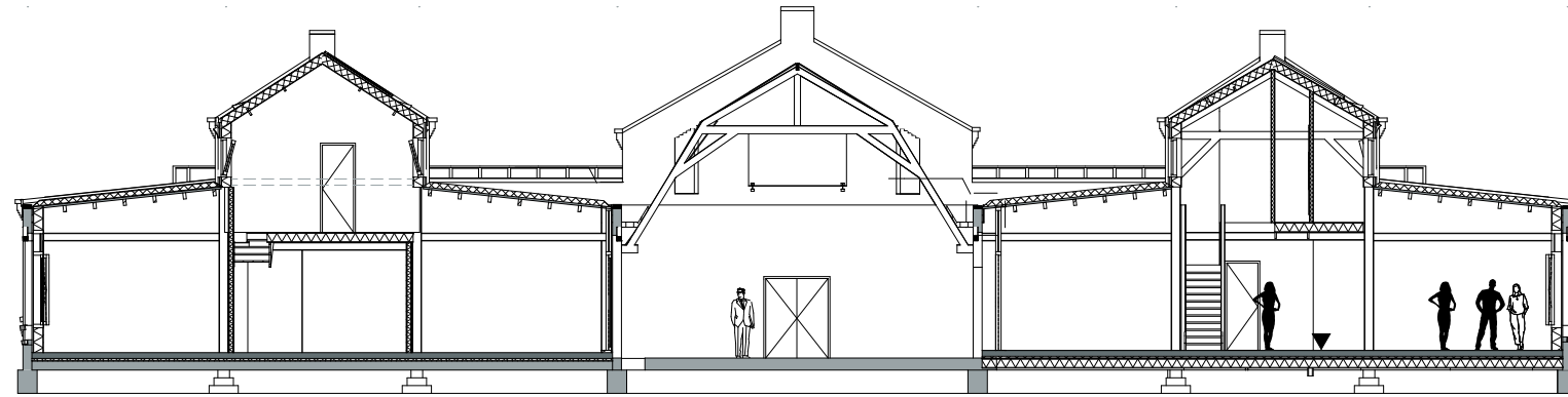
Doorsnede CC
