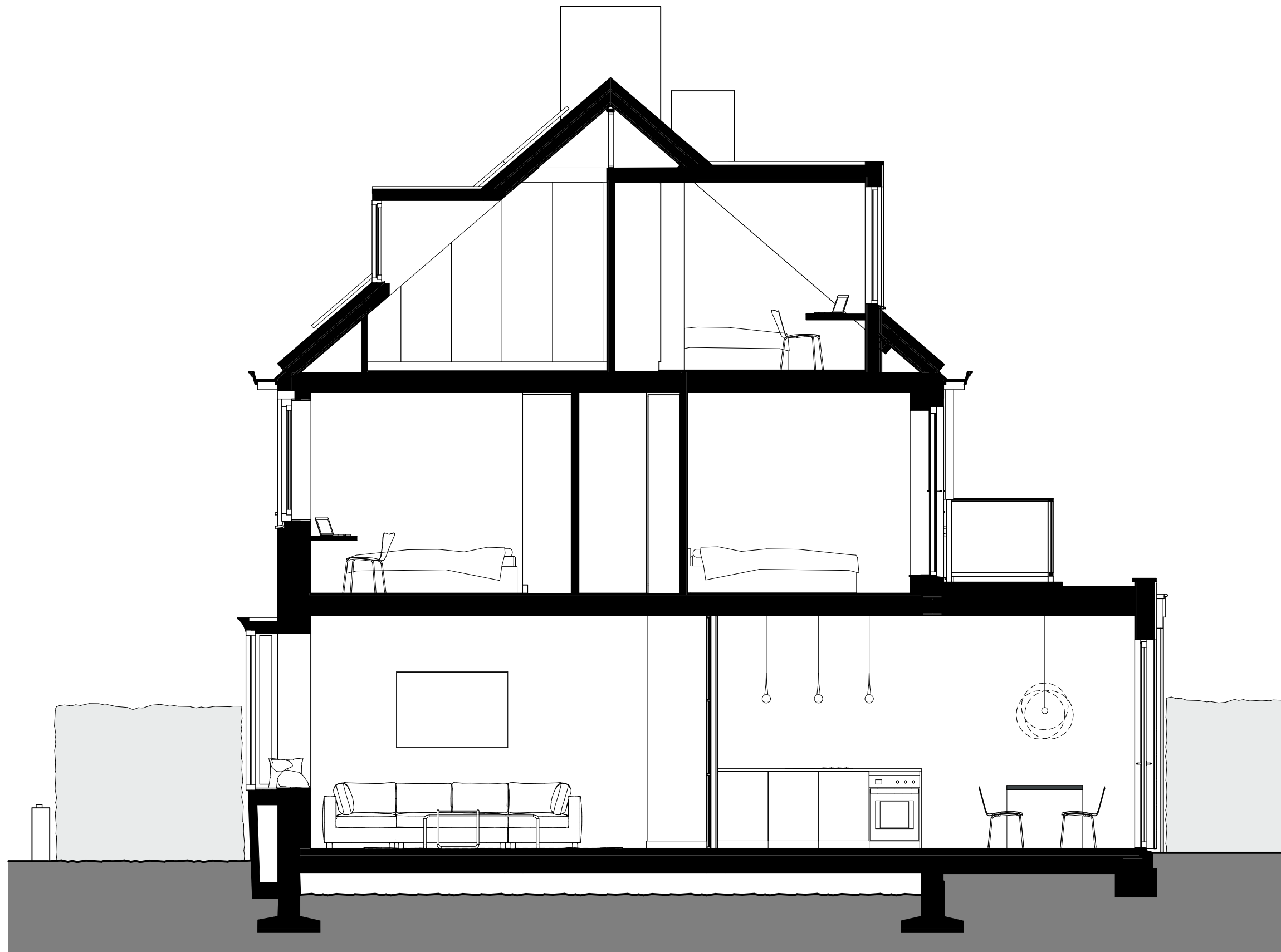
doorsnede
